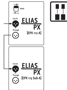
Anschluss-Schema Standard-System
