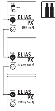
Anschluss-Schema Extension-Setup
